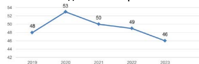
Динамика пожаров
